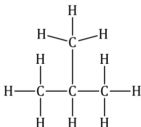
iso-Butane
